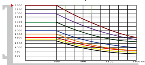
Остаточная грузоподъемность в зависимости от центра тяжести
