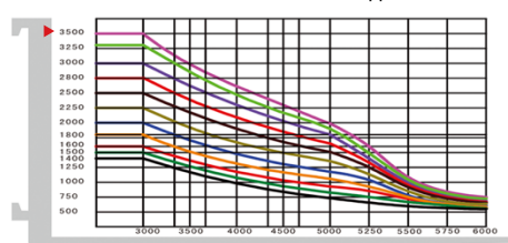
Остаточная грузоподъемность в зависимости от высоты подъема
