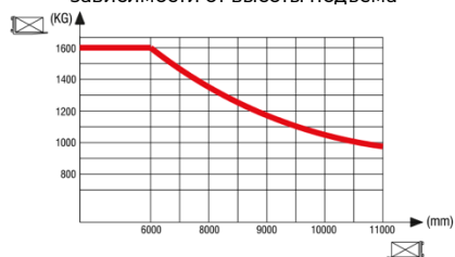
Остаточная грузоподъемность в зависимости от высоты подъема
